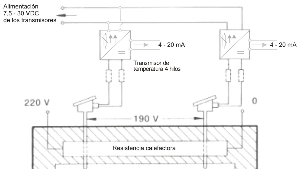
Figura 5 : Conexión de dos sensores de temperatura mediante transmisores de temperatura 4 hilos con aislación galvánica
