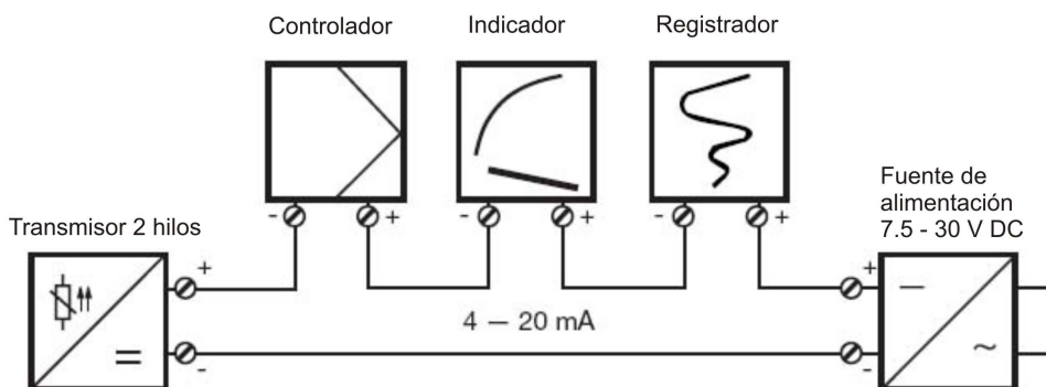
Figura 10: Diagrama de conexión para un transmisor de temperatura de dos hilos con fuente de alimentación
