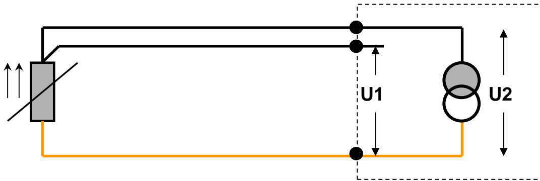
Figura 11. Conexión 3 hilos
