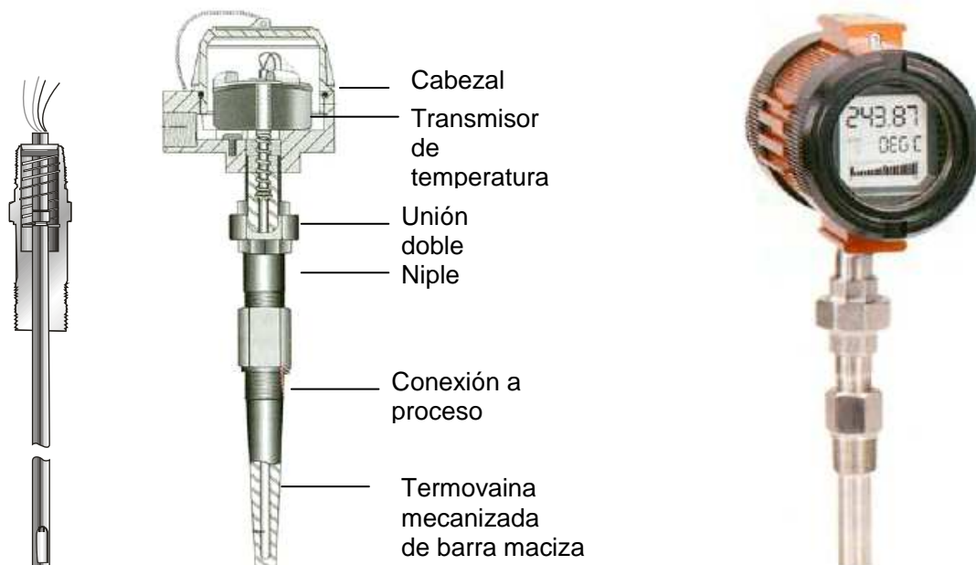
Figura 9: Montaje de sensor "Spring loaded" tipo ASTM
