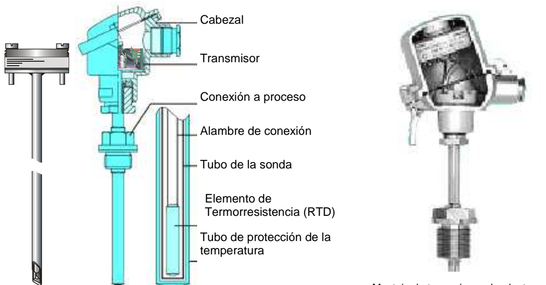
Figura 7: Montaje intercambiable sonda tipo DIN con transmisor
