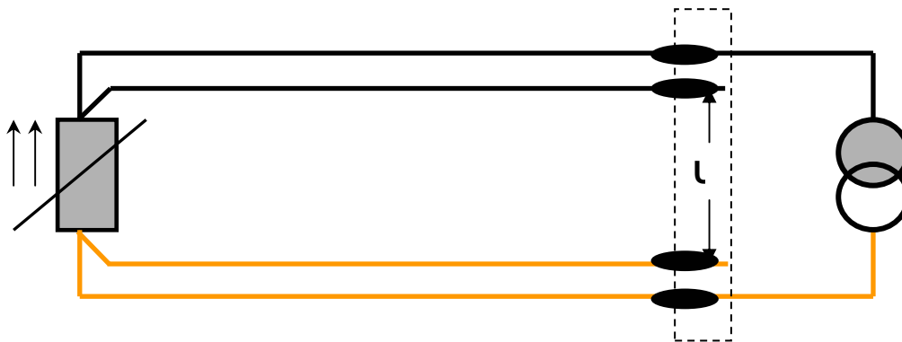
Figura 12. Conexión 4 hilos.
