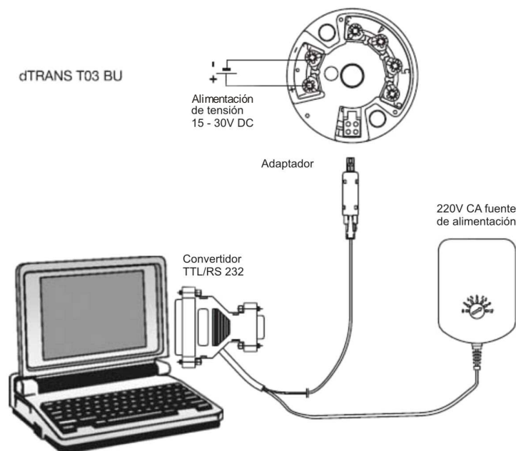
Figura 8: Configuración de un transmisor de temperatura JUMO dTRANS T03 BU mediante software dedicado y LapTop
